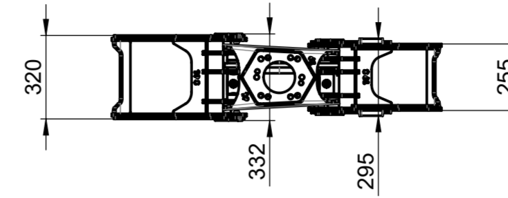
BG019/S Holzgreifer 105 kg
