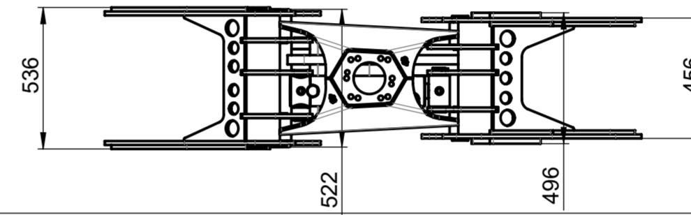
BG043/R4 Reissiggreifer 310 kg
