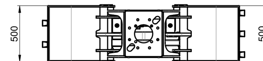
BEHA BUG 7-9 290 kg
