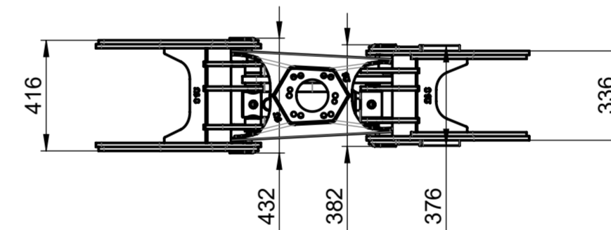
BG026/SR4 Reissiggreifer 195 kg
