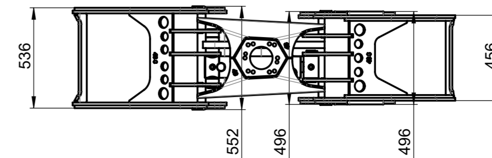
BG043/S Holzgreifer 375 kg
