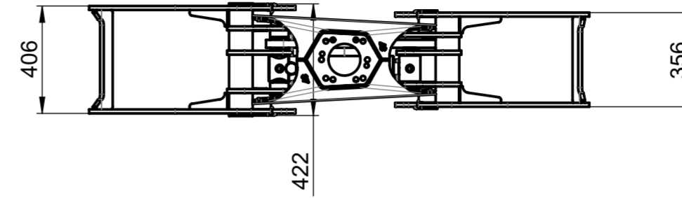
BG037 Holzgreifer 185 kg
