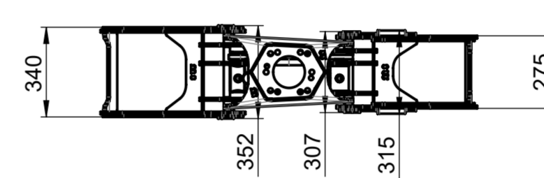
BG022 S Holzgreifer 130 kg
