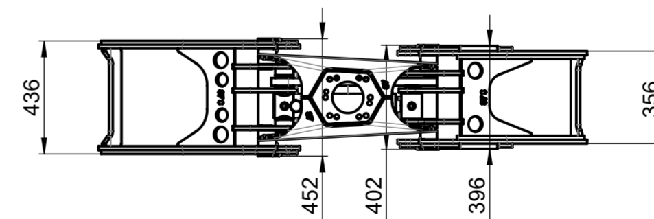
BG037/S Holzgreifer 275 kg
