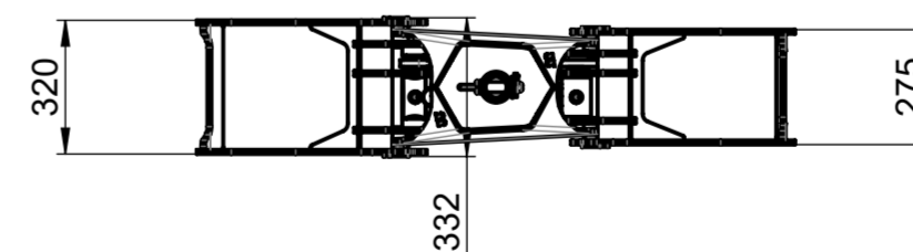
BG026 Holzgreifer 145 kg
