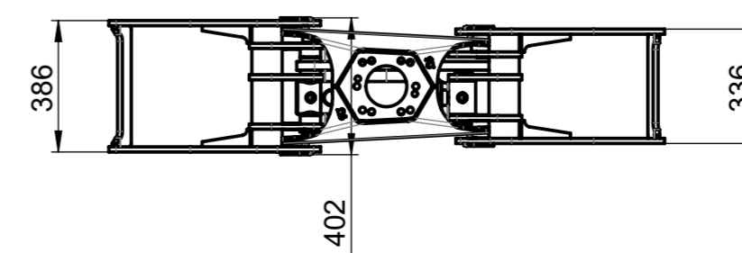
BG026 Holzgreifer 145 kg
