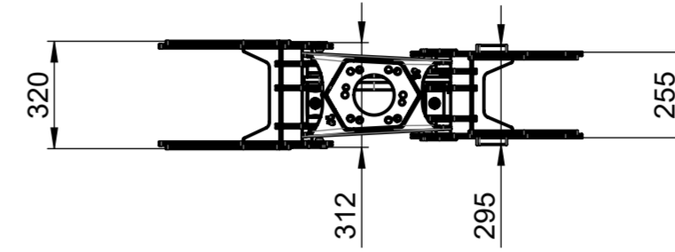
BG019/R4 Reissiggreifer 80 kg
