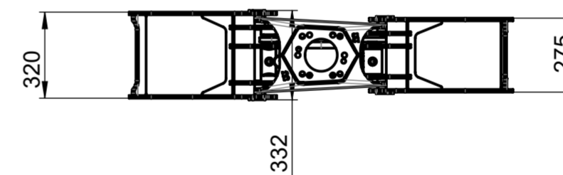
BG022/50 Holzgreifer 105 kg
