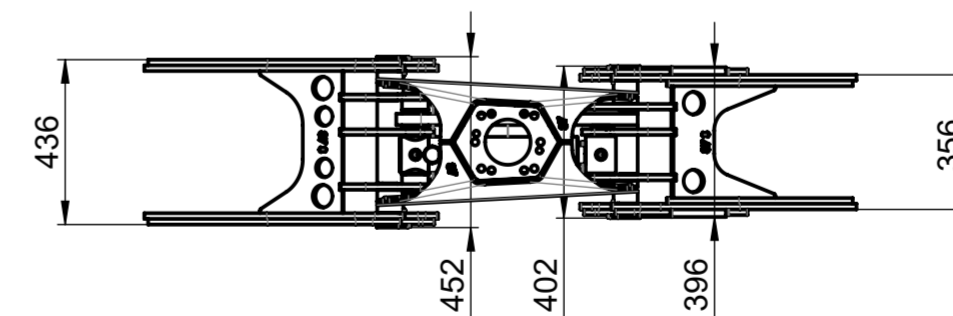
BG037/SR4 Reissiggreifer 265 kg
