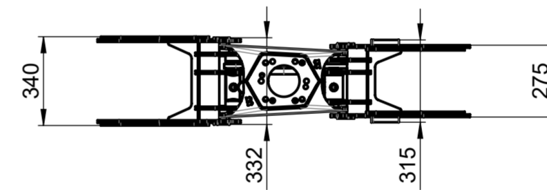
BG022/R4 Reissiggreifer 105 kg
