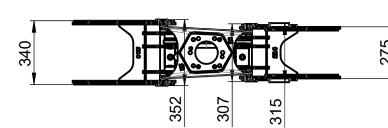
BG022 SR4 Reissiggreifer 130 kg
