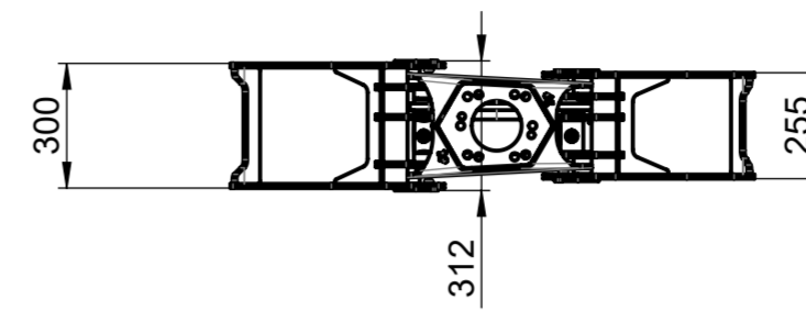
BG019 Holzgreifer 75 kg
