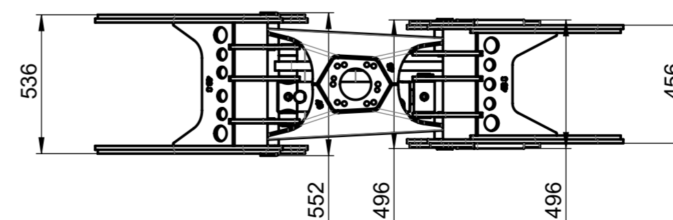
BG043/SR4 Reissiggreifer 360 kg
