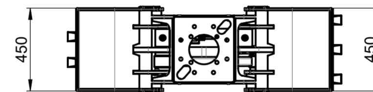
BEHA BUG 5-7 230 kg
