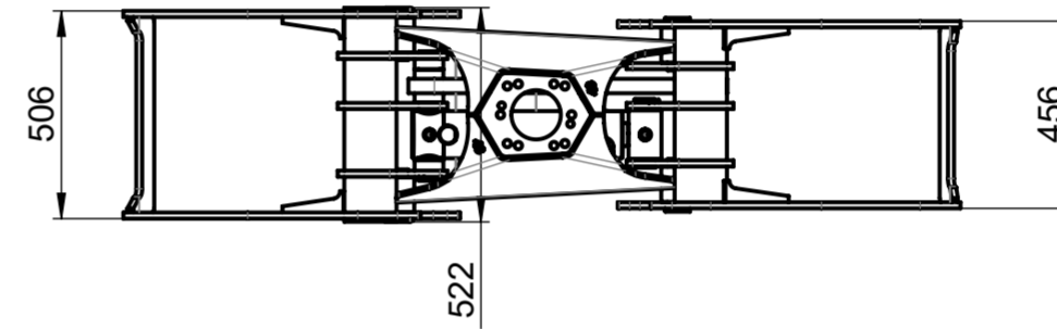
BG043 Holzgreifer 275 kg
