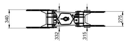
BG022/R4/50 Reissiggreifer 110 kg
