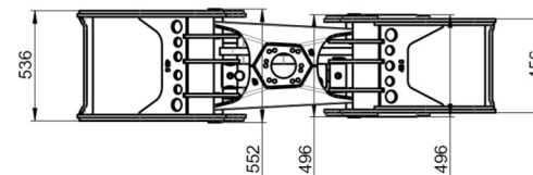
BG043/S Holzgreifer 375 kg
