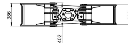
BG026 Holzgreifer 145 kg
