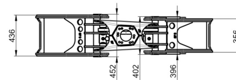
BG037/S Holzgreifer 275 kg
