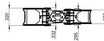
BG019/S Holzgreifer 105 kg
