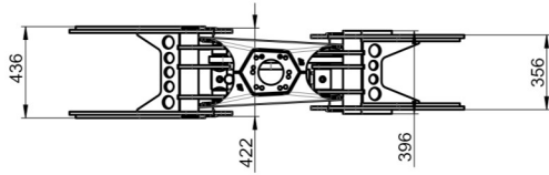
BG037/R4 Reissiggreifer 230 kg
