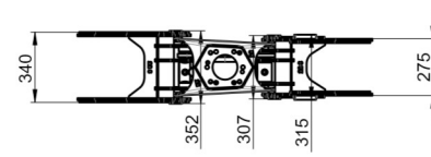
BG026/SR4 Reissiggreifer 195 kg
