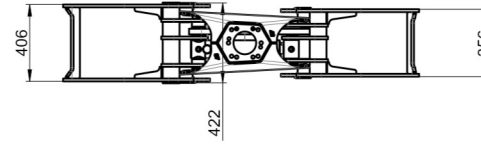
BG043 Holzgreifer 275 kg
