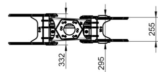
BG022 SR4 Reissiggreifer 130 kg
