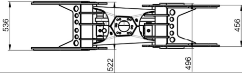
BG043/R4 Reissiggreifer 310 kg
