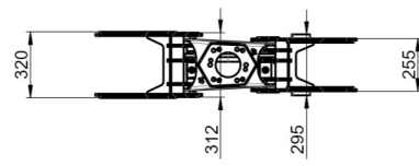
BG019/R4 Reissiggreifer 80 kg
