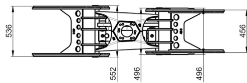
BG043/SR4 Reissiggreifer 360 kg
