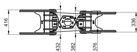
BG026/SR4 Reissiggreifer 195 kg
