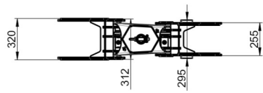
BG019/R4/50 Reissiggreifer 85 kg
