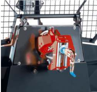
Seilausstoß mit leistungstarkem Hydraulikmotor
