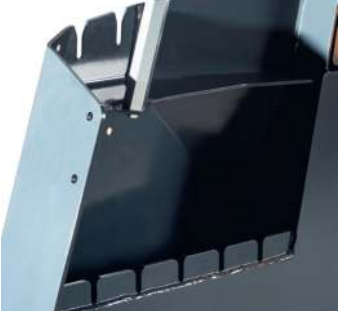
Große Ablagen vorne an der Winde, damit der Schmutz von Schlepperrädern nicht die Ketten und das andere Zubehör erreicht.
